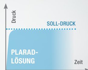
Plarad-Hydraulikaggregate mit Spannzylinder-Modus
