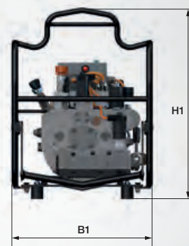
Plarad-Hydraulikaggregate mit Spannzylinder-Modus
